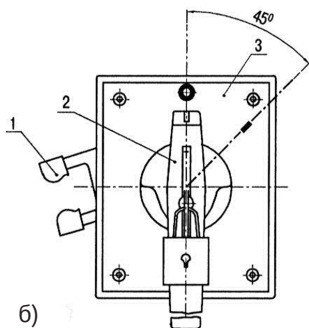
Рисунок Б.14 – Запирающее устройство в положении «Отключено» а) выключателей стационарного исполнения, б) выключателей с ручным дистанционным приводом
