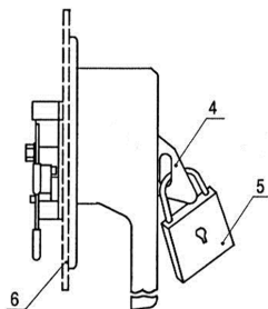
Рисунок Б.14 – Запирающее устройство в положении «Отключено» а) выключателей стационарного исполнения, б) выключателей с ручным дистанционным приводом
