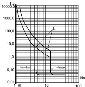
Рисунок А.6 - Временно-токовые характеристики выключателей на ток 160 А, 200 А, 250 А
