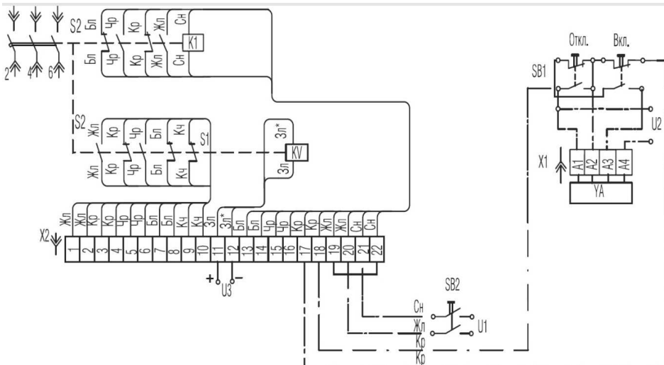
Рисунок Б.3 - Схема электрическая принципиальная выключателей выдвижного исполнения с дополнительными сборочными единицами
