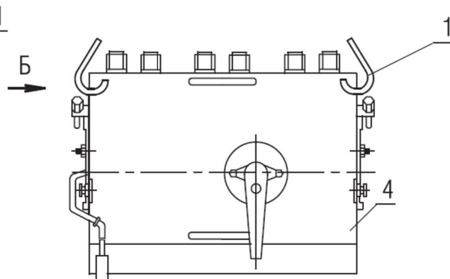
Выключатель без выдвижного устройства
