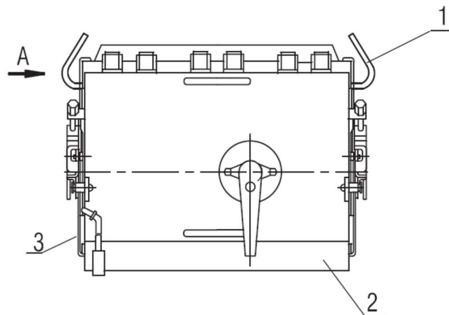
Выключатель в выдвижном устройстве
