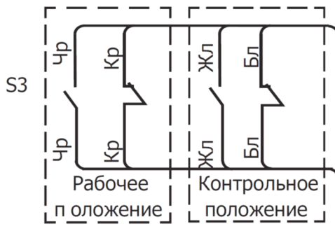
Рисунок Б.8 - Схема электрическая принципиальная контактов сигнализации рабочего и контрольного положений выключателя выдвижного исполнения
