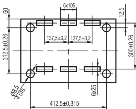
Рисунок 1 - Отверстия в панели для установки выключателей (вид спереди)
