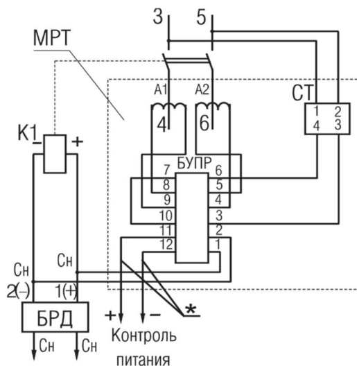
Стационарное исполнение
