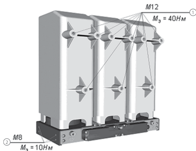
Рис. 14. Точки крепления коммутационных модулей ISM15_Shell_2, ISM15_Shell_FT2
