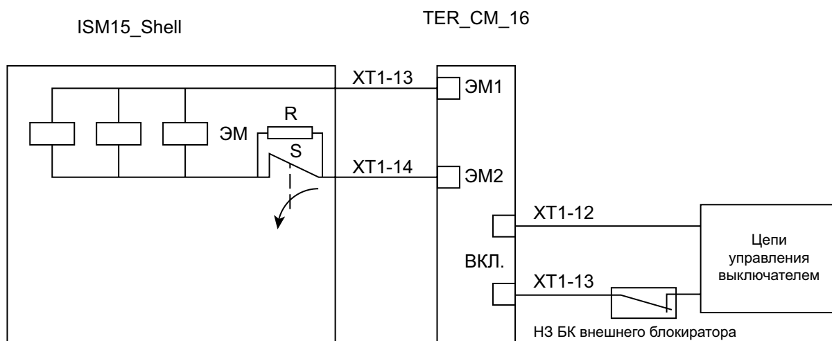
Рис. 43. Электрическая блокировка ISM15_Shell с TER_CM_16
