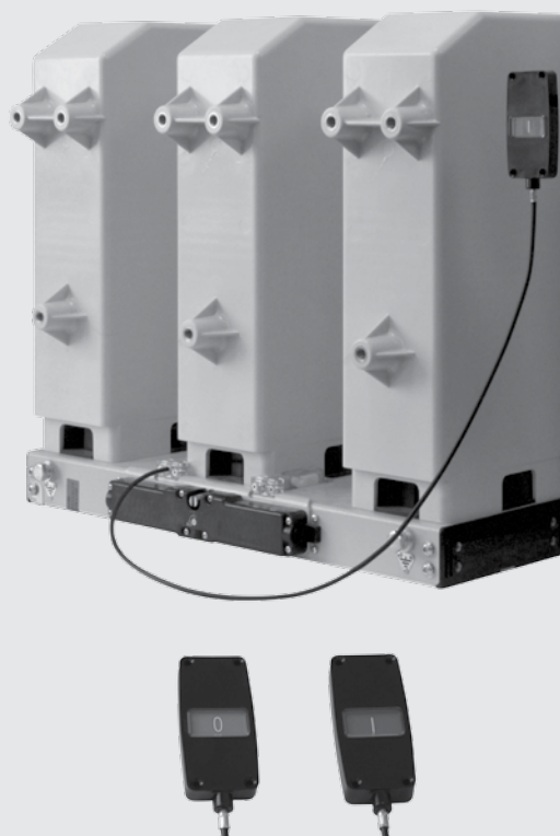
Рис. 11. Индикатор положения главных контактов
