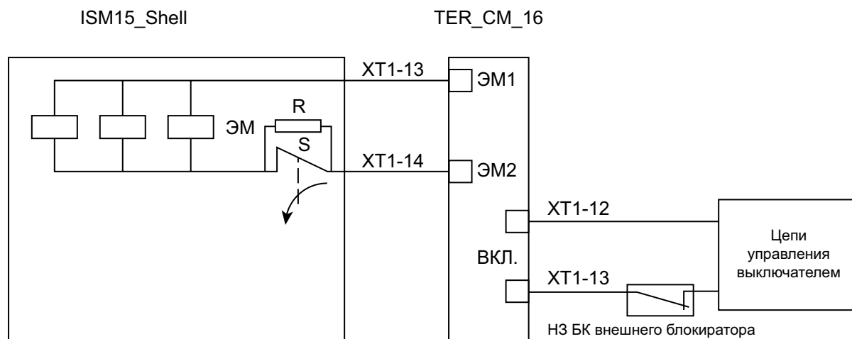
Рис. 42. Электрическая блокировка ISM15_Shell_2 с БУ/TEL-12А, БУ/TEL-21-00 и ISM15_Shell_FT2 с CM_1501_01(4)
