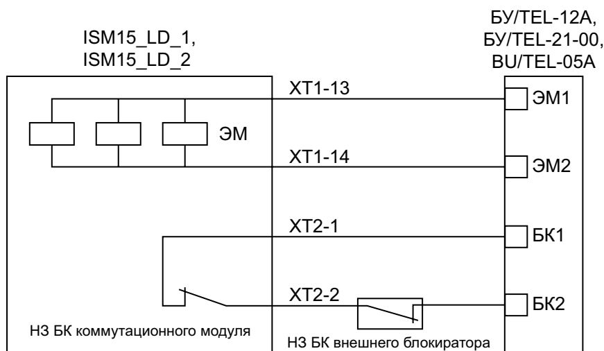
Рис. 40. Электрическая блокировка ISM15_LD_1, ISM15_LD_2 с БУ/TEL-12А, БУ/TEL-21-00, БУ/TEL-05А
