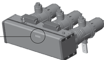
Рис. 46. Индикатор положения главных контактов ISM15_LD_1(45), ISM15_LD_1(46).
