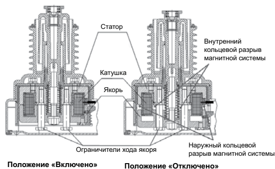
Рис. 10. Двухразрывный привод коммутационных модулей, ISM15_Shell_2, ISM15_Shell_FT2
