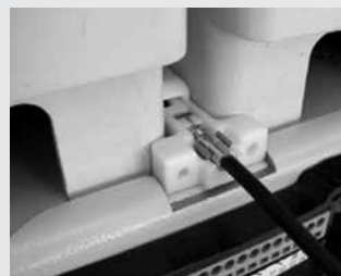
Рис. 48. Установка троса
