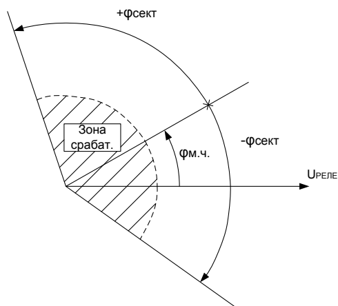
Рис. 2.1. Максимальная токовая защита: а - функциональная схема МТЗ; б - функциональная схема ПОН; в - область срабатывания органа направления мощности и «Сириус-2-С», а также в расширенном варианте с наличием ПОН и направленностью – ряд других терминалов (см. таблицу 2.1.).
