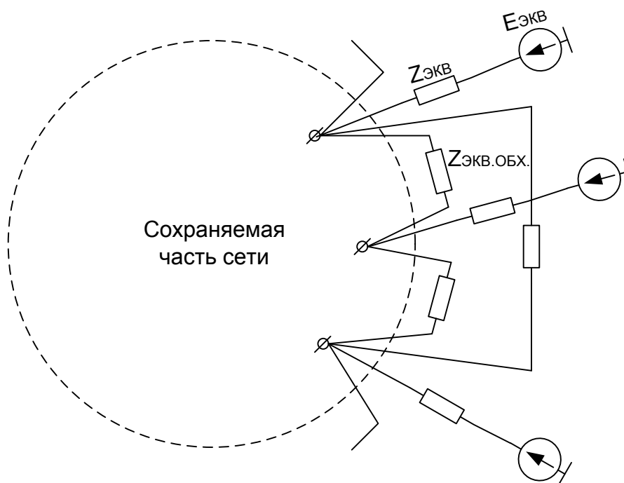
Рис. 1.7. Эквивалентирование сети
