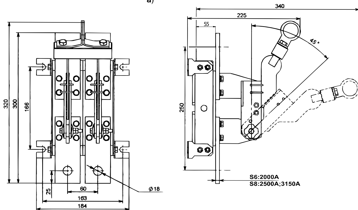
Рис. 45. Разъединитель PE19 однополюсный а) PE19-44(45; 46)-11110-00 УХЛЗ с центральной рукояткой; б) PE19-44(45; 46)-11190-00 УХЛЗ с центральным рычагом для управления штангой
