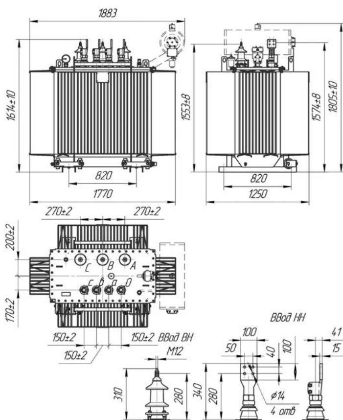
ТМГ-СЭЩ(ТМ-СЭЩ)-1250/10-11
