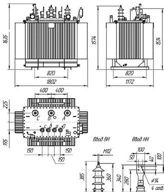
ТМГ-СЭЩ-1000/20(15)-11
