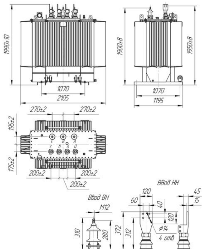
ТМГ-СЭЩ-1600/10-12
