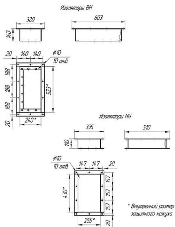
Фланец ТМ(Г)Ф-СЭ Щ-400/10-11
