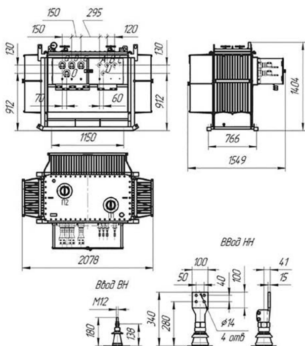
ТМПНГ-СЭЩ-800-11
